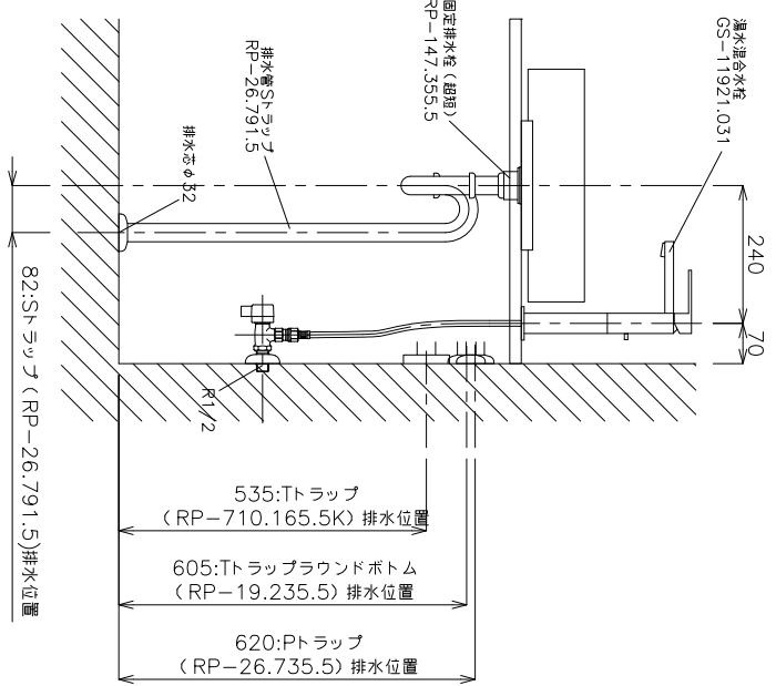
側面図
