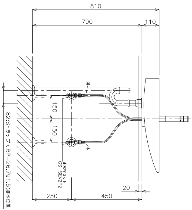
立面図
