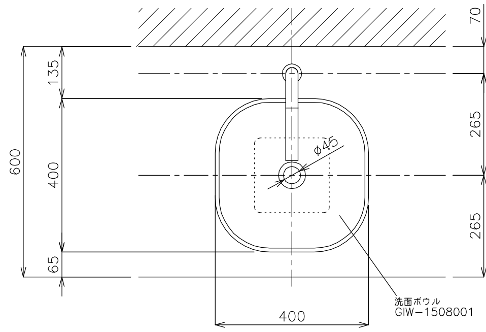
洗面ボウル GIW-1508001 平面図
