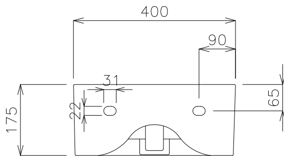
背図
