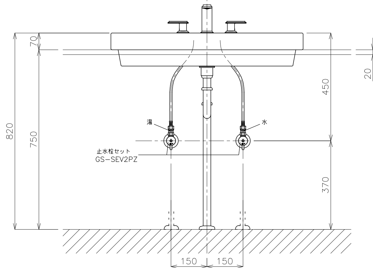
立面図
