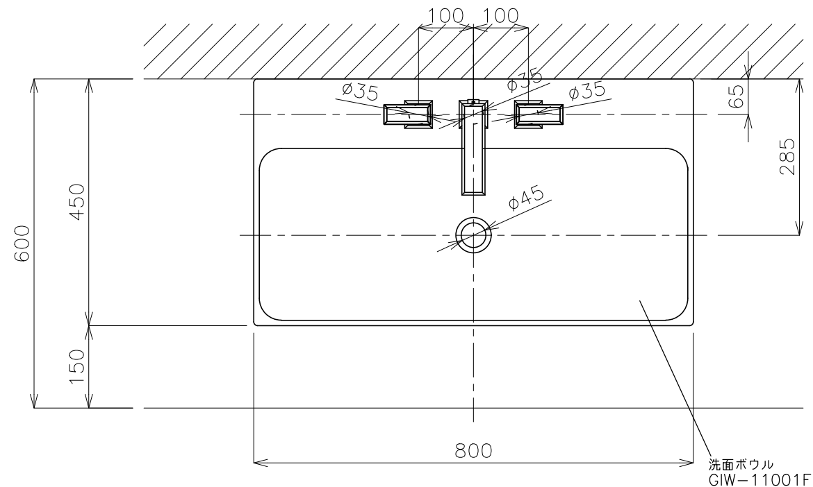
平面図
