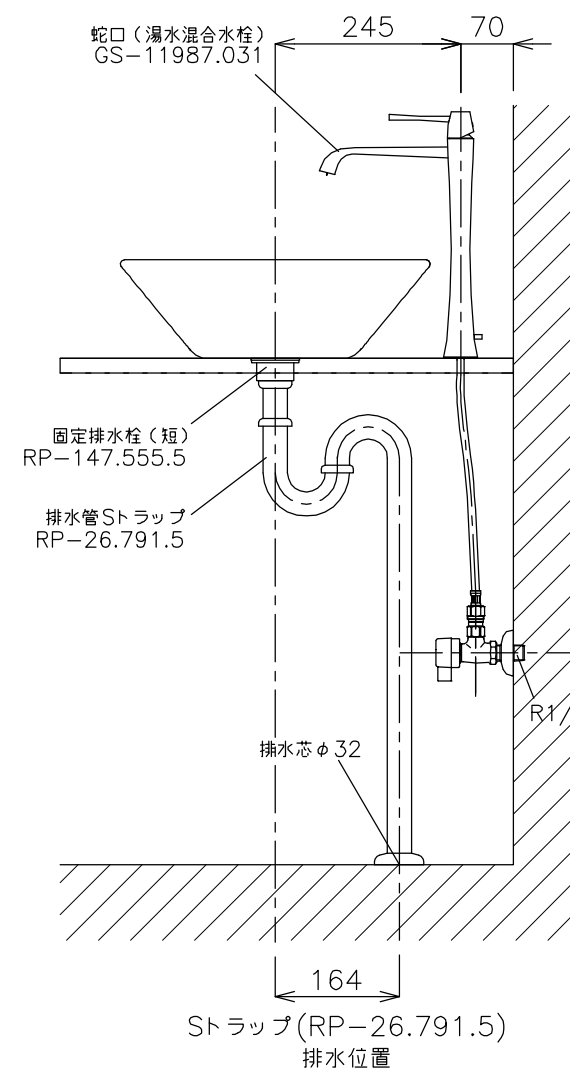
側面図
