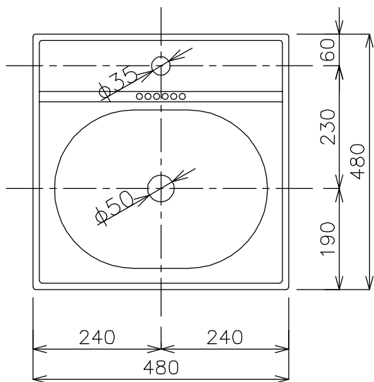
平面図
