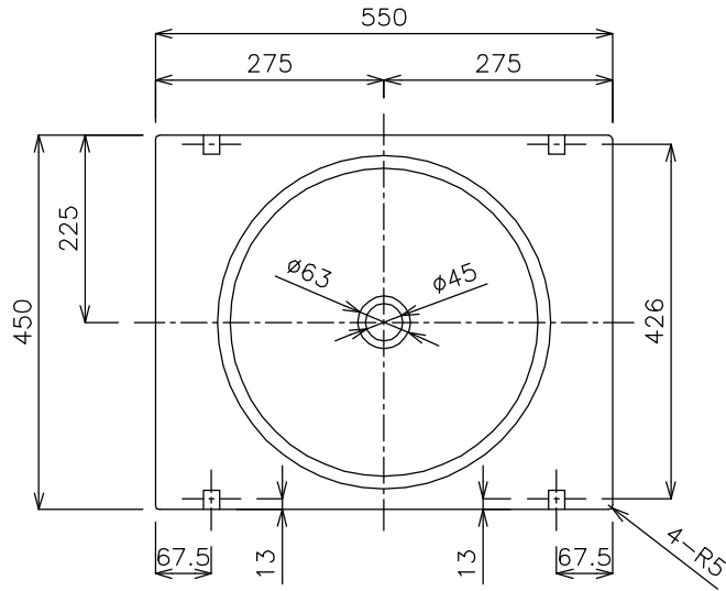
平面図
