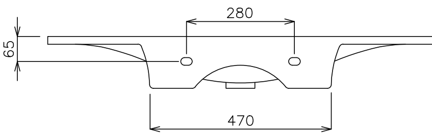
立面図
