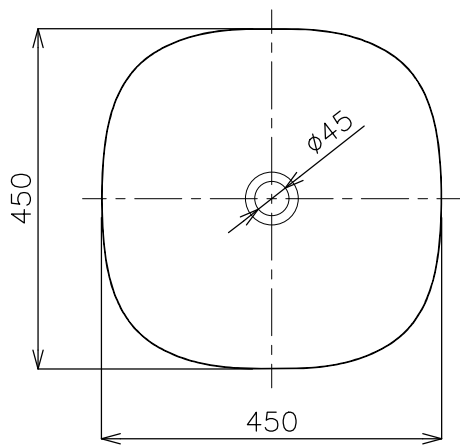
平面図
