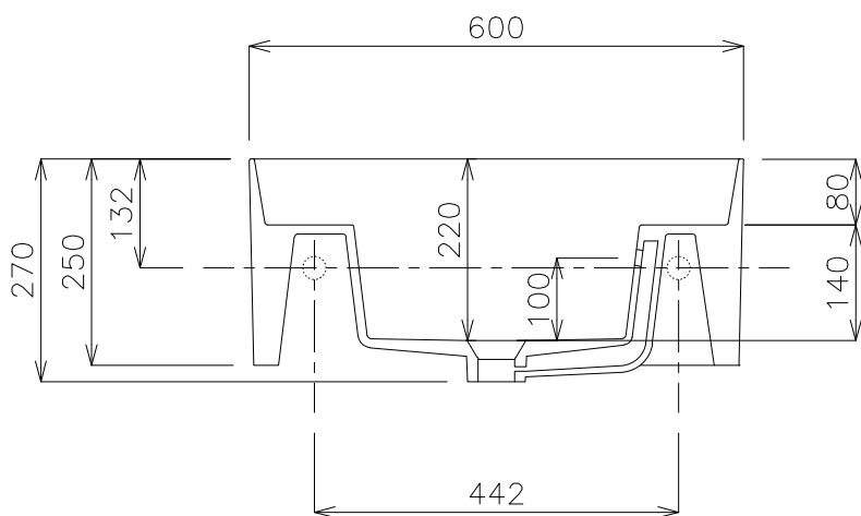
断面 A-A
